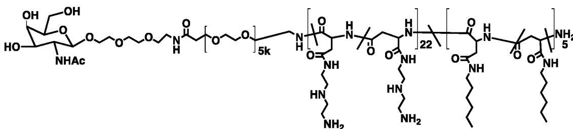
GalNAc-PEG5K-pASP(DET)-C6
