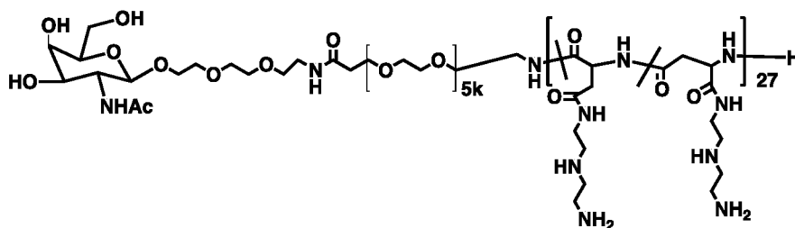
GalNAc-PEG5K-pASP(DET)
